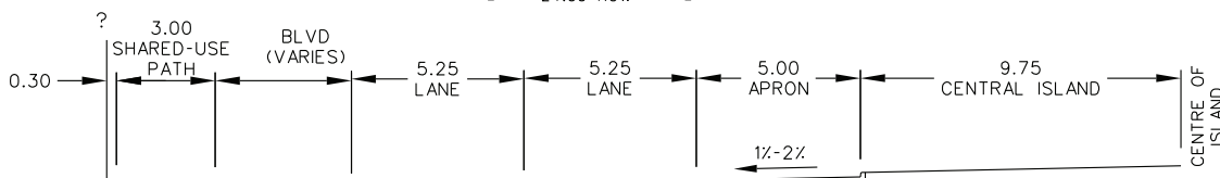
SECTION A-A
